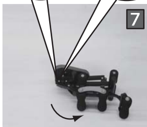
7 リアレッグ側の[2]ロックピンを外し、リアレッグを折りたたみます。外した[2]ロックピンは、紛失しないように元のリアレッグ用固定穴に差し込んでください。
