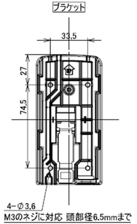
取付参考図
